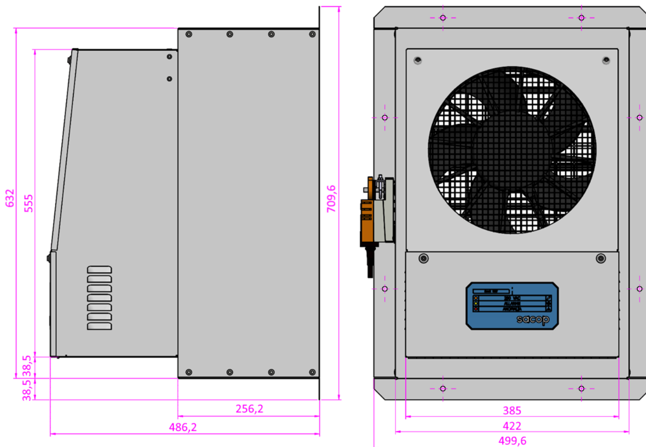
Figura 7 - Misure unità Black EVO con box serranda
