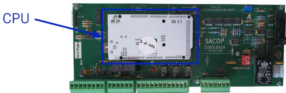
Figura 49 - Indicazione CPU su circuito stampato scheda elettronica E003.0014
