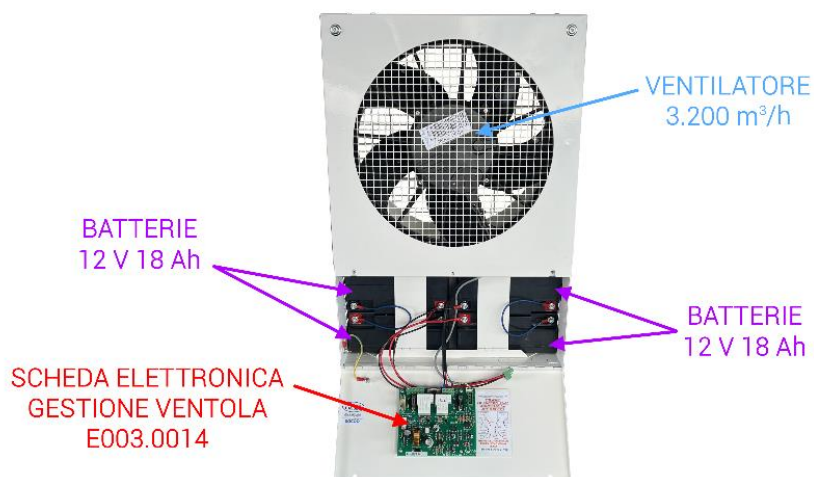
Figura 4 - Componenti principali unità Black EVO 3.2
