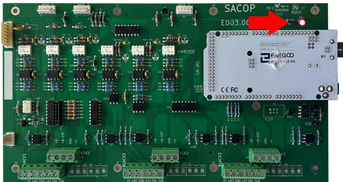
Figura 13 - Led ROSSO denominato DL5 su scheda elettronica Multimaster E003.0021
