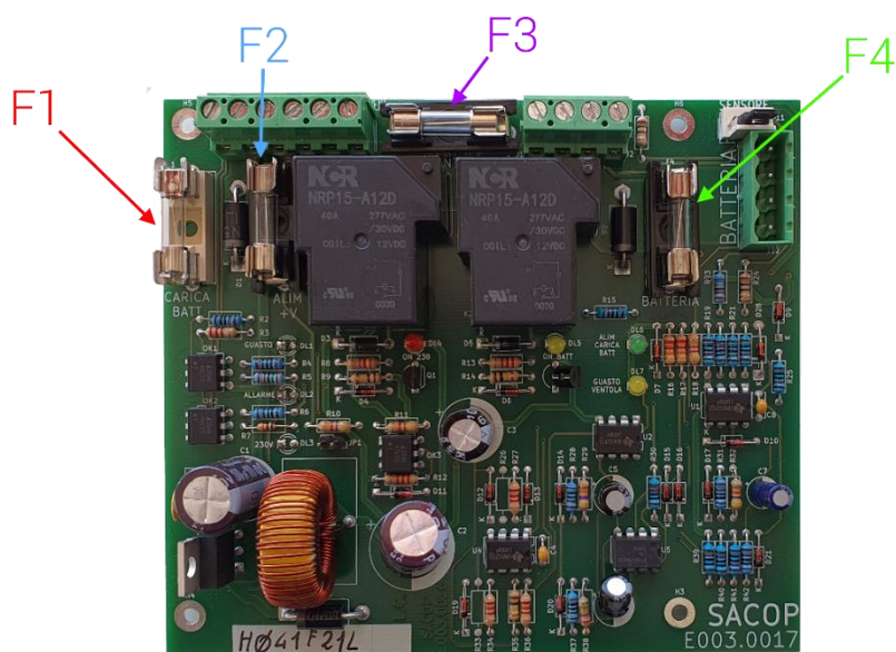
Figura 53 - Posizionamento fusibili su scheda elettronica gestione ventola E003.0017 unità Black EVO
