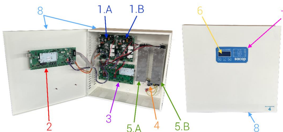
Figura 45 - Indicazione ricambi unità Multimaster 4
