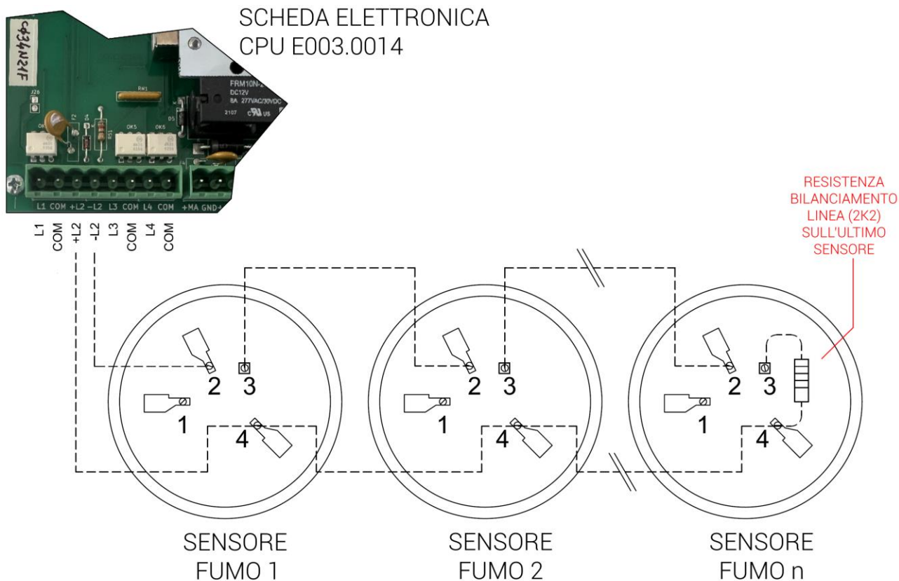
Figura 66 - Schema di collegamento rilevatori fumo
