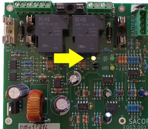
Figura 18 - Led GIALLO denominato DL5 ON BATT
