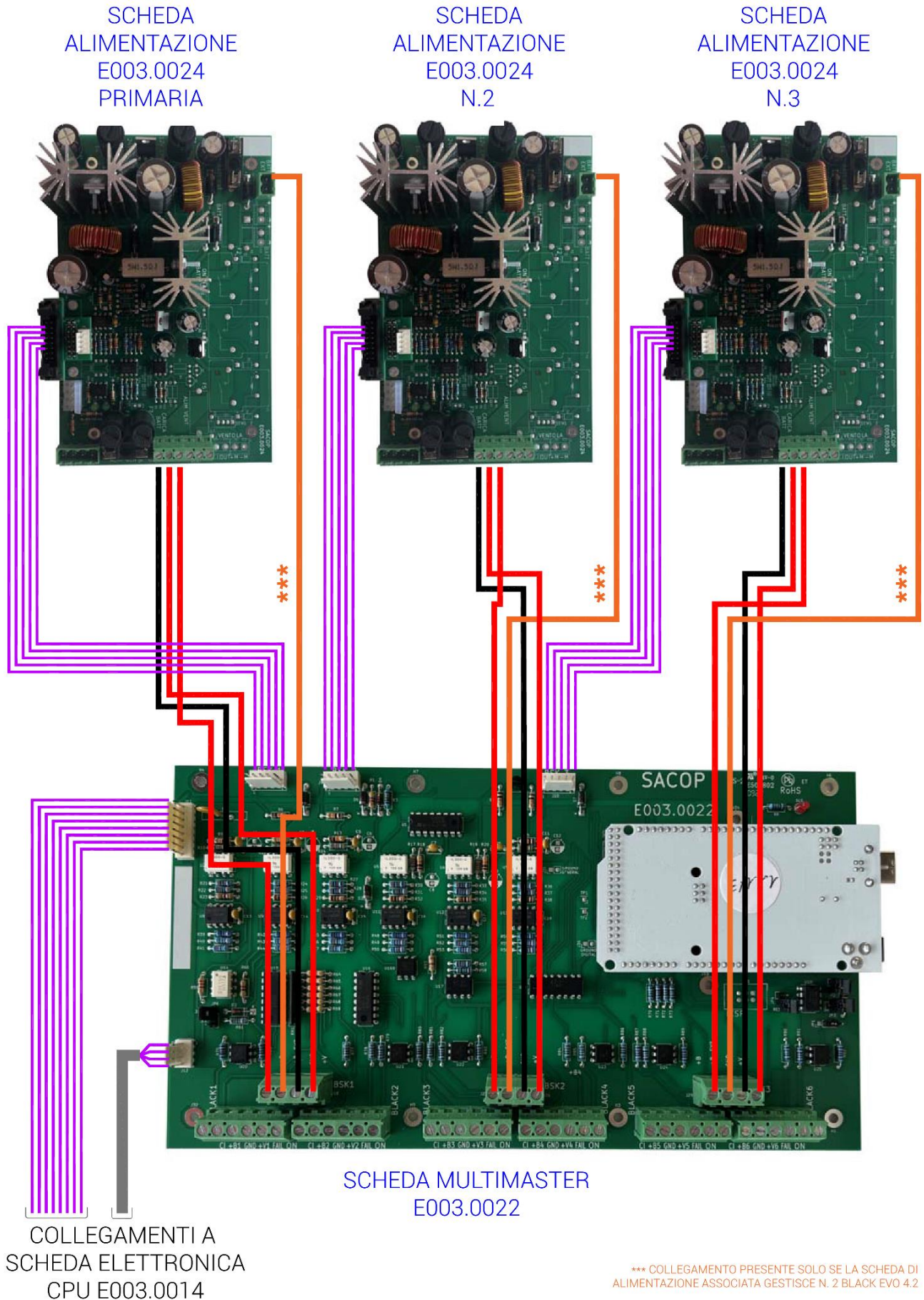
Figura 58 - Schema collegamento elettrico tra scheda elettronica Multimaster E003.0022 e le schede di alimentazione E003.0024 nella configurazione massima (n. 6 Black EVO 4.2)
