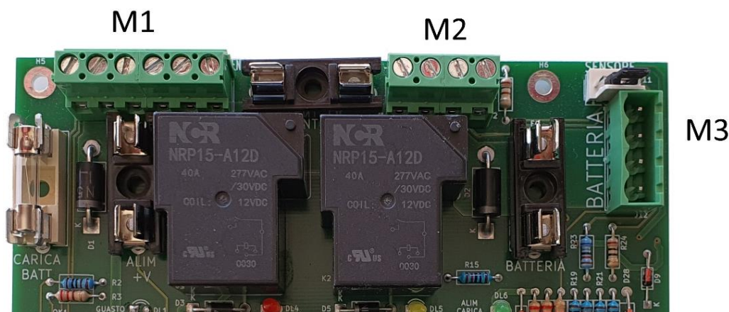
Figura 16 - Morsettiere scheda elettronica gestione ventola E003.0017
