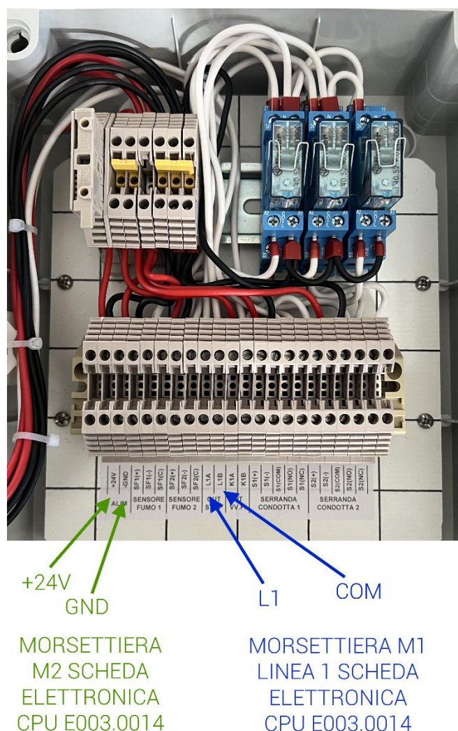
Figura 42 - Collegamento elettrico del quadro di interfaccia serrande e pulsante VV.F.
