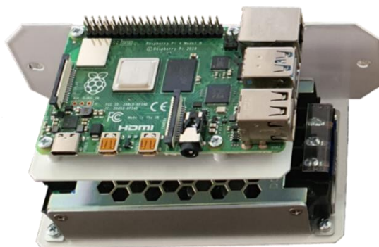
Figura 29 - Scheda di comunicazione WiFi / Bluetooth MBL-99-12 per Sacop Connect
