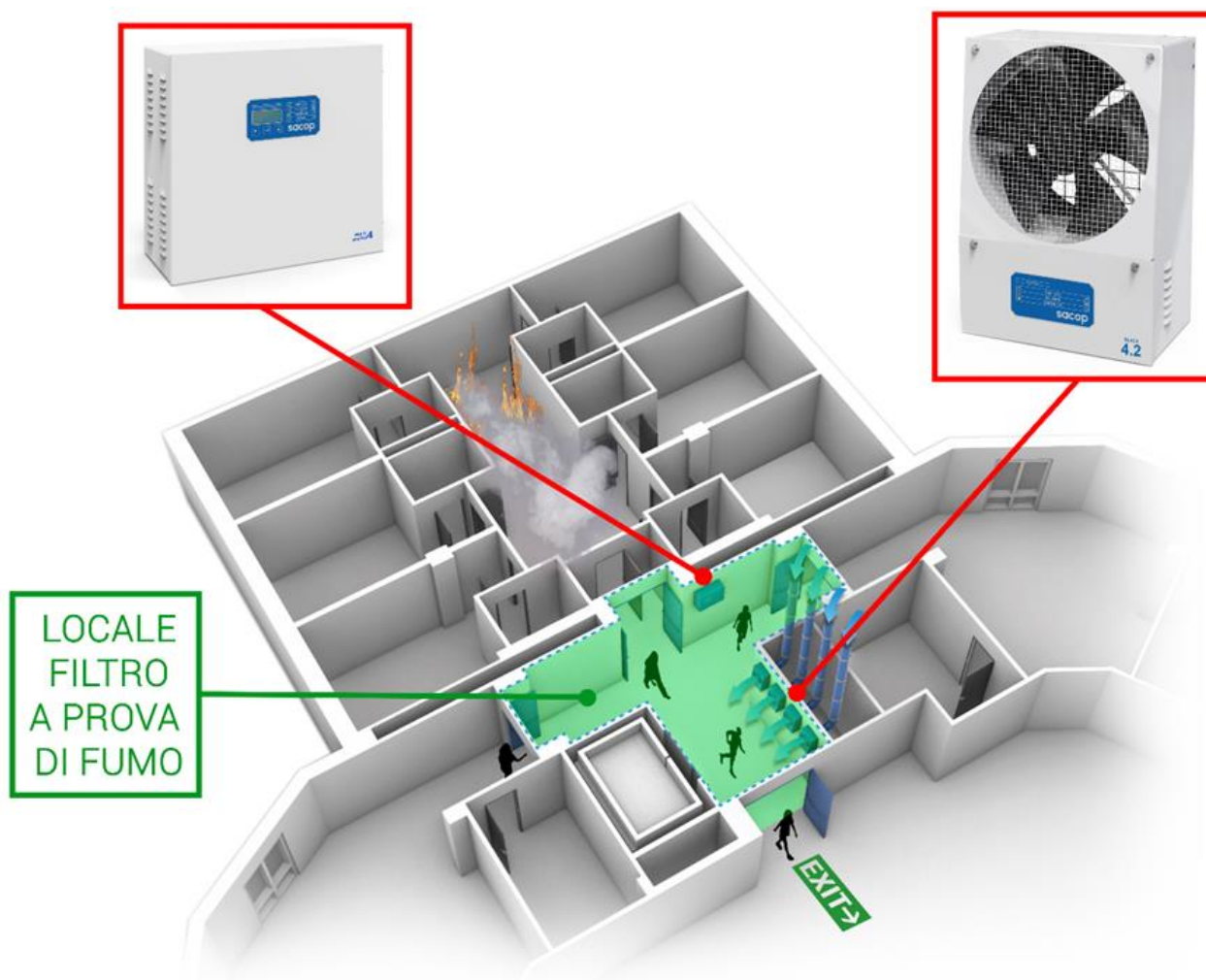
Figura 1 - Esempio di installazione di un sistema di sovrappressione Multimaster Black EVO per "filtro a prova di fumo"
