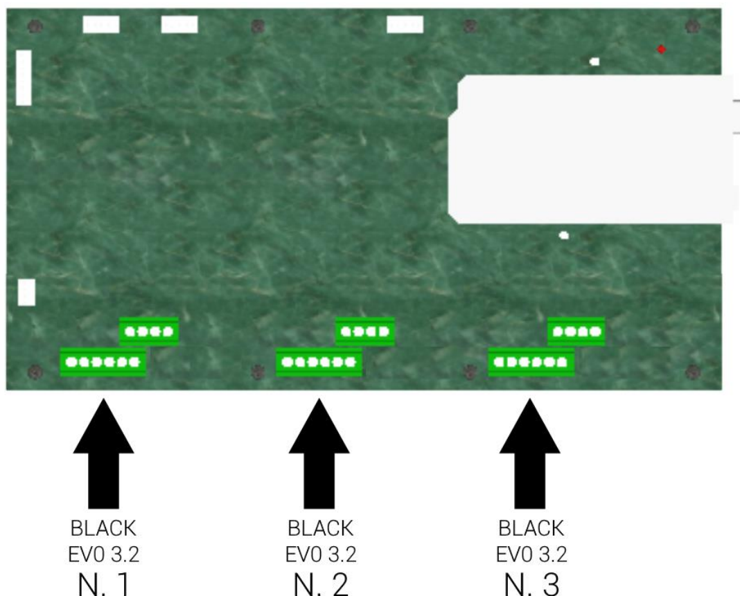
Figura 23 - Schema di collegamento Black EVO 3.2 (fino a 3 unità)
