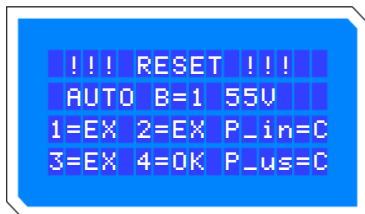
Visualizzazione display in "Reset" per modello con Black EVO 4.2
