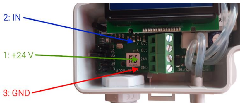
Figura 40 - Collegamento elettrico pressostato differenziale
