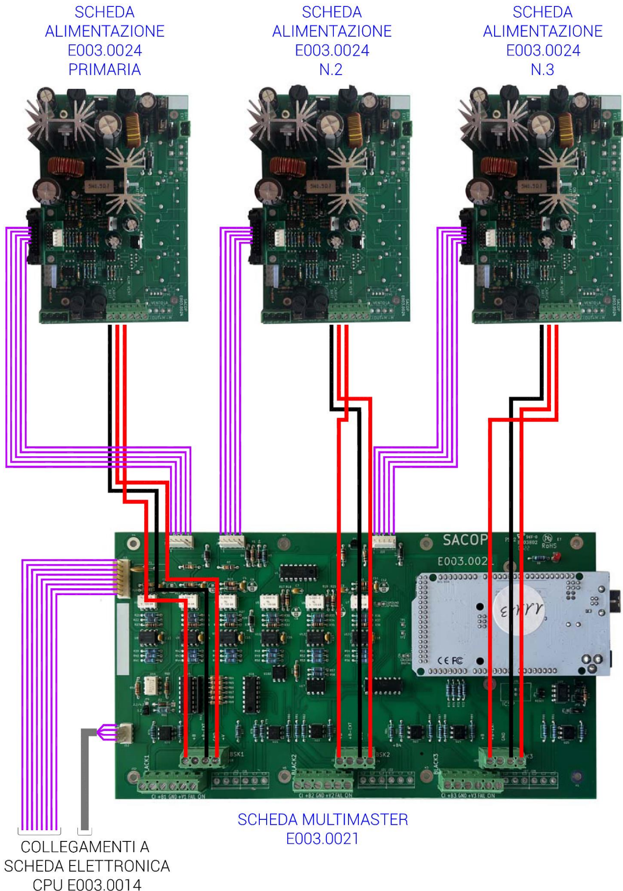
Figura 57 - Schema collegamento elettrico tra scheda elettronica Multimaster E003.0021 e le schede di alimentazione E003.0024 nella configurazione massima (n. 3 Black EVO 3.2)
