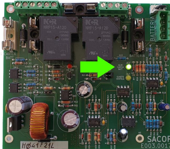
Figura 19 - Led VERDE denominato DL6 ALIM CARICA BATT
