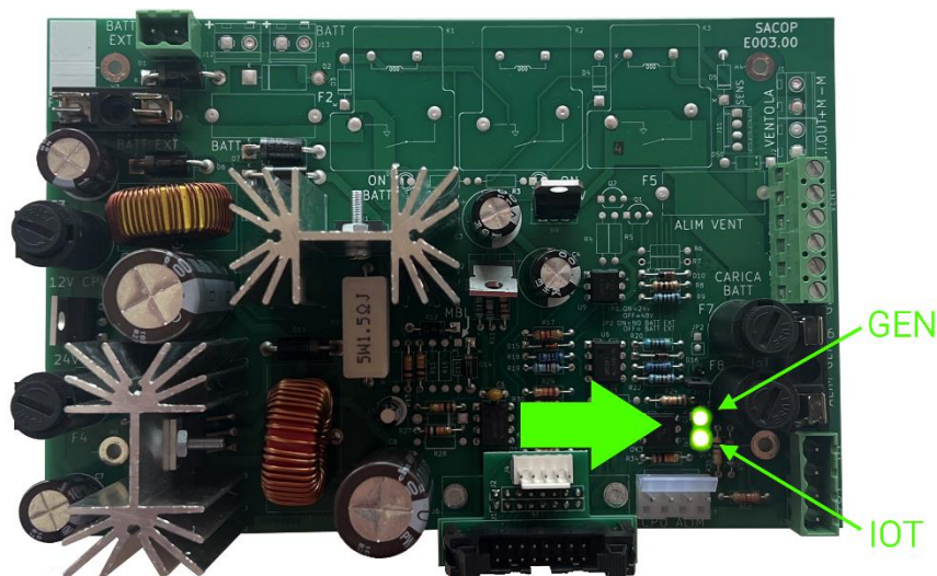
Figura 8 - Led VERDI denominati GEN e IOT su scheda elettronica di alimentazione E003.0024
