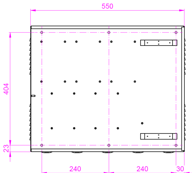
Figura 36 - Quote fori unità Multimaster 6
