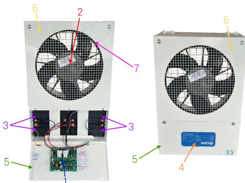
Figura 47 - Indicazione ricambi unità Black EVO 3.2
