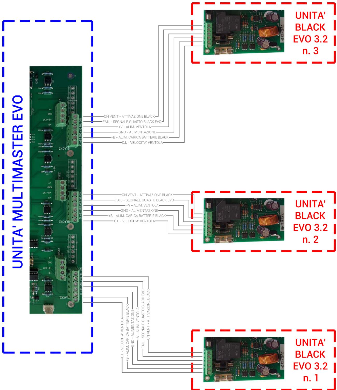
Figura 55 - Schema collegamento elettrico tra scheda elettronica Multimaster E003.0021 / E003.0022 (unità Multimaster) e schede elettroniche gestione ventola E003.0017 (unità Black EVO 3.2)
