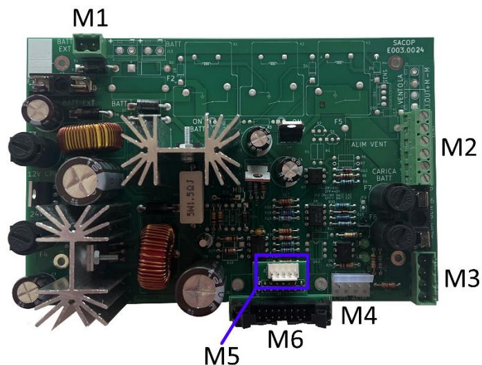
Figura 7 - Morsettiere scheda elettronica di alimentazione E003.0024
