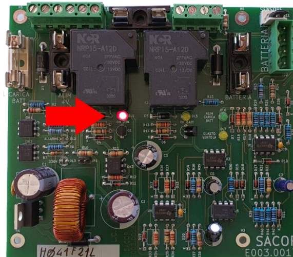
Figura 17 - Led ROSSO denominato DL4 ON 230
