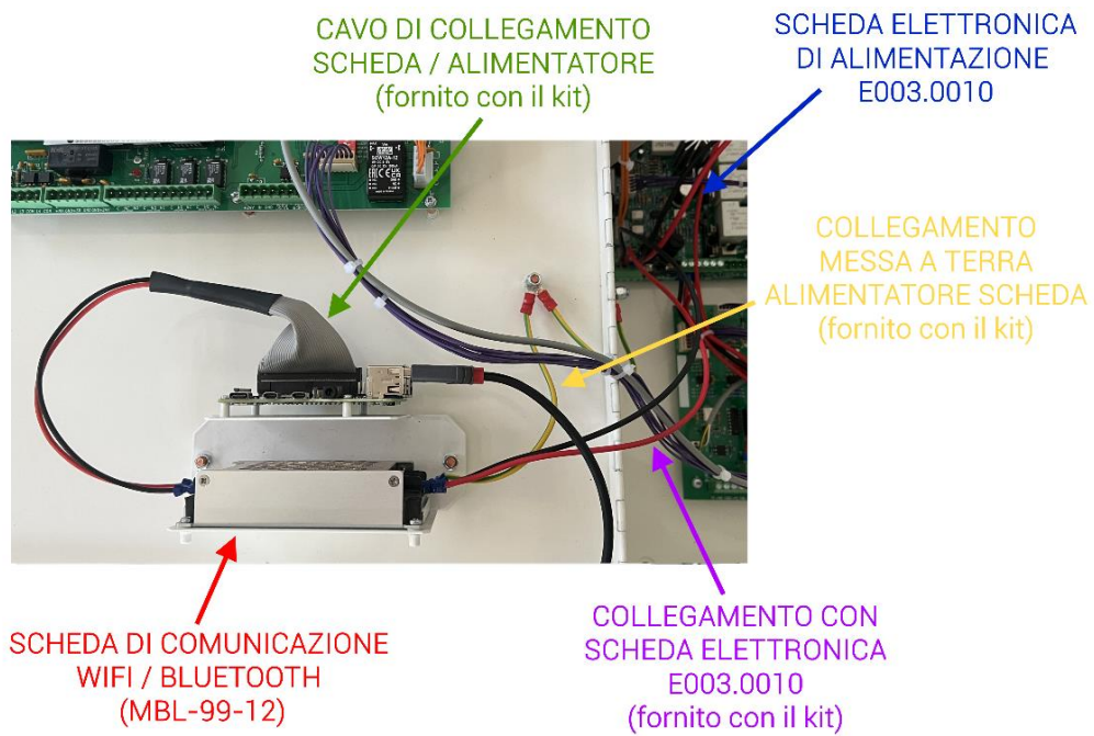
Figura 30 - Modalità di installazione scheda di comunicazione WiFi / Bluetooth MBL-99-12 per Sacop Connect
