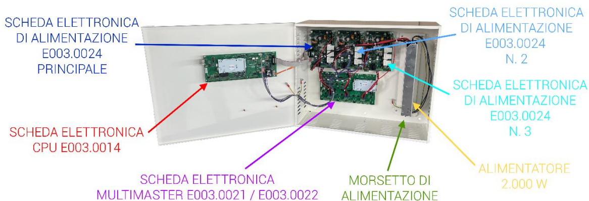
Figura 3 - Componenti principali unità Multimaster 6
