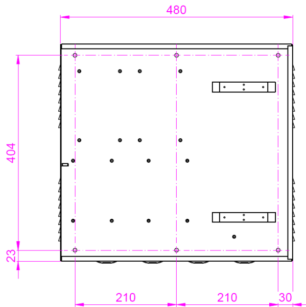
Figura 35 - Quote fori unità Multimaster 4
