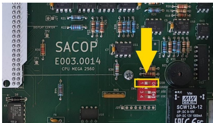
Figura 33 - Dip switch 1 su scheda elettronica CPU E003.0014 (unità Multimaster) per silenziare il BUZZER
