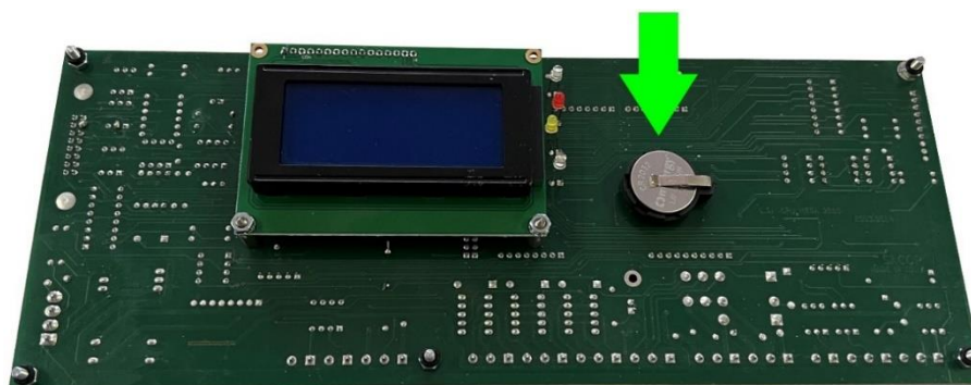
Figura 11 - Batteria del tipo CR2032 su scheda E003.0014 da sostituire ogni 3 anni
