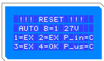
Visualizzazione display in "Reset" per modello con Black EVO 3.2
