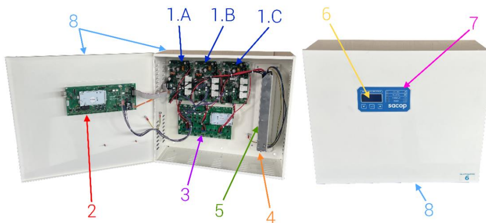
Figura 46 - Indicazione ricambi unità Multimaster 6
