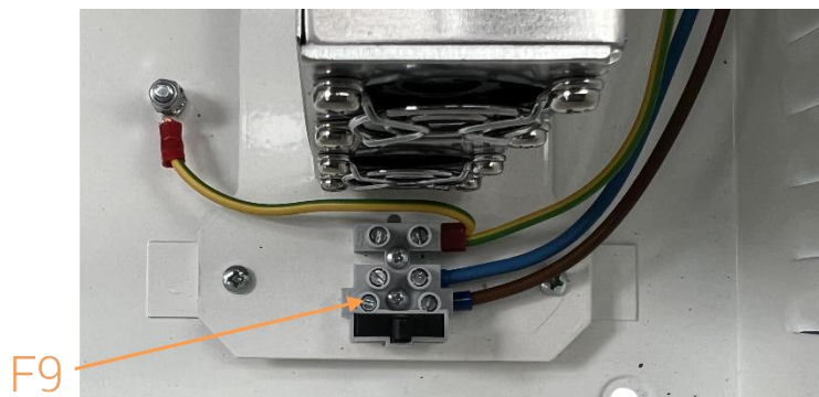
Figura 52 - Fusibile su morsetto di alimentazione unità Multimaster 6
