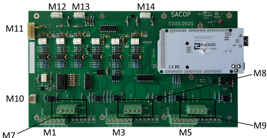
Figura 12 - Morsettiera scheda elettronica Multimaster E003.0021
