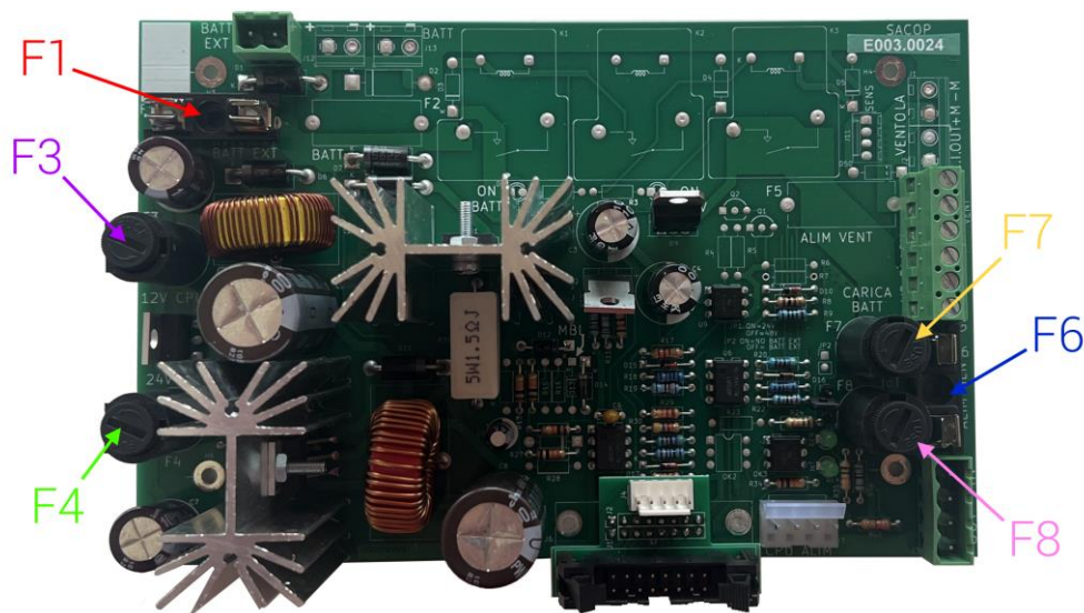
Figura 50 - Posizionamento fusibili su schede elettroniche di alimentazione E003.0024 unità Multimaster
