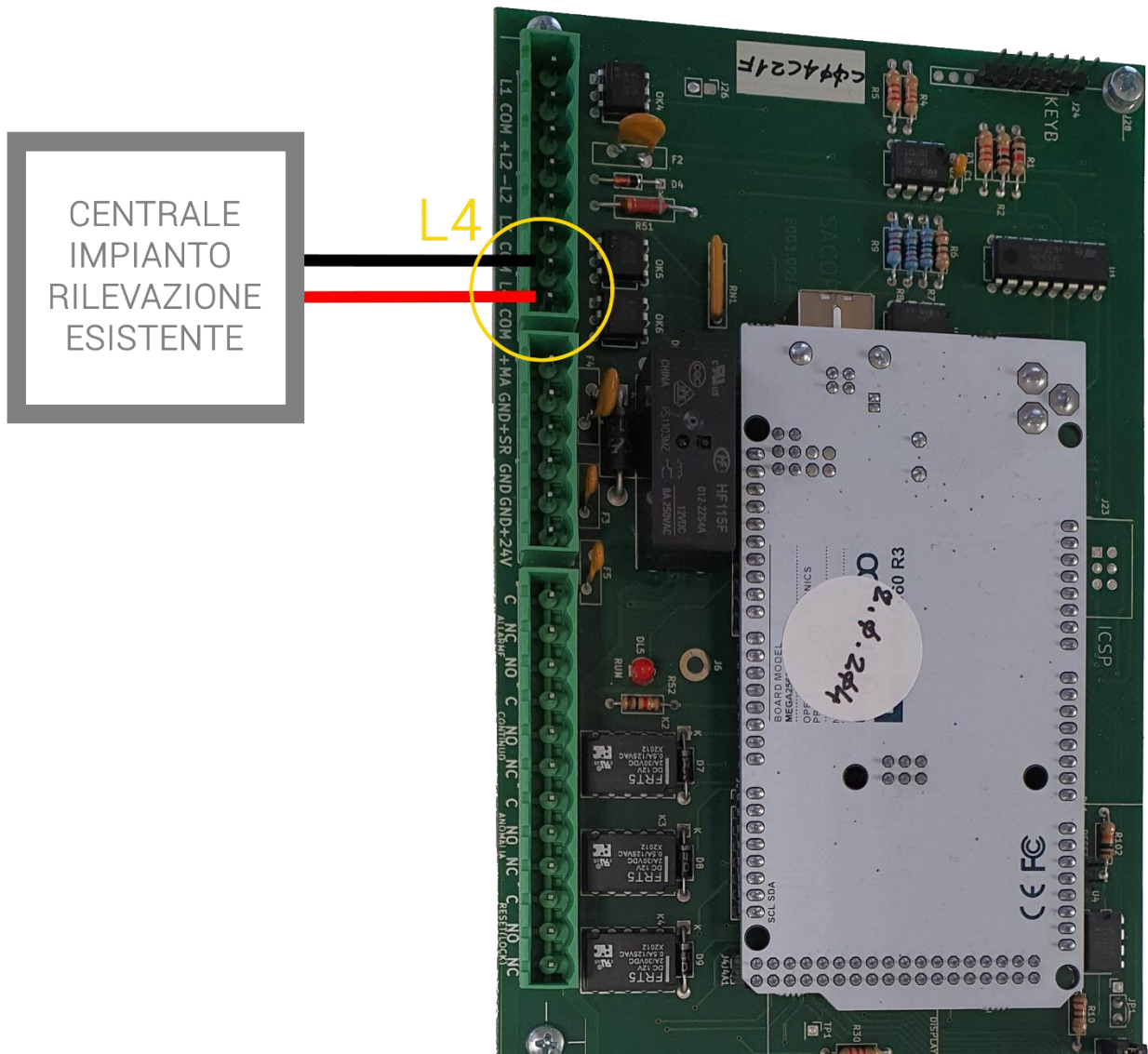
Figura 54 - Schema collegamento elettrico impianto rilevazione incendio esistente scheda elettronica CPU E003.0014
