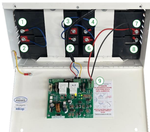
Figura 38 - Foto interna unità Black EVO 4.2 e sequenza operazioni per collegamento cavi batterie
