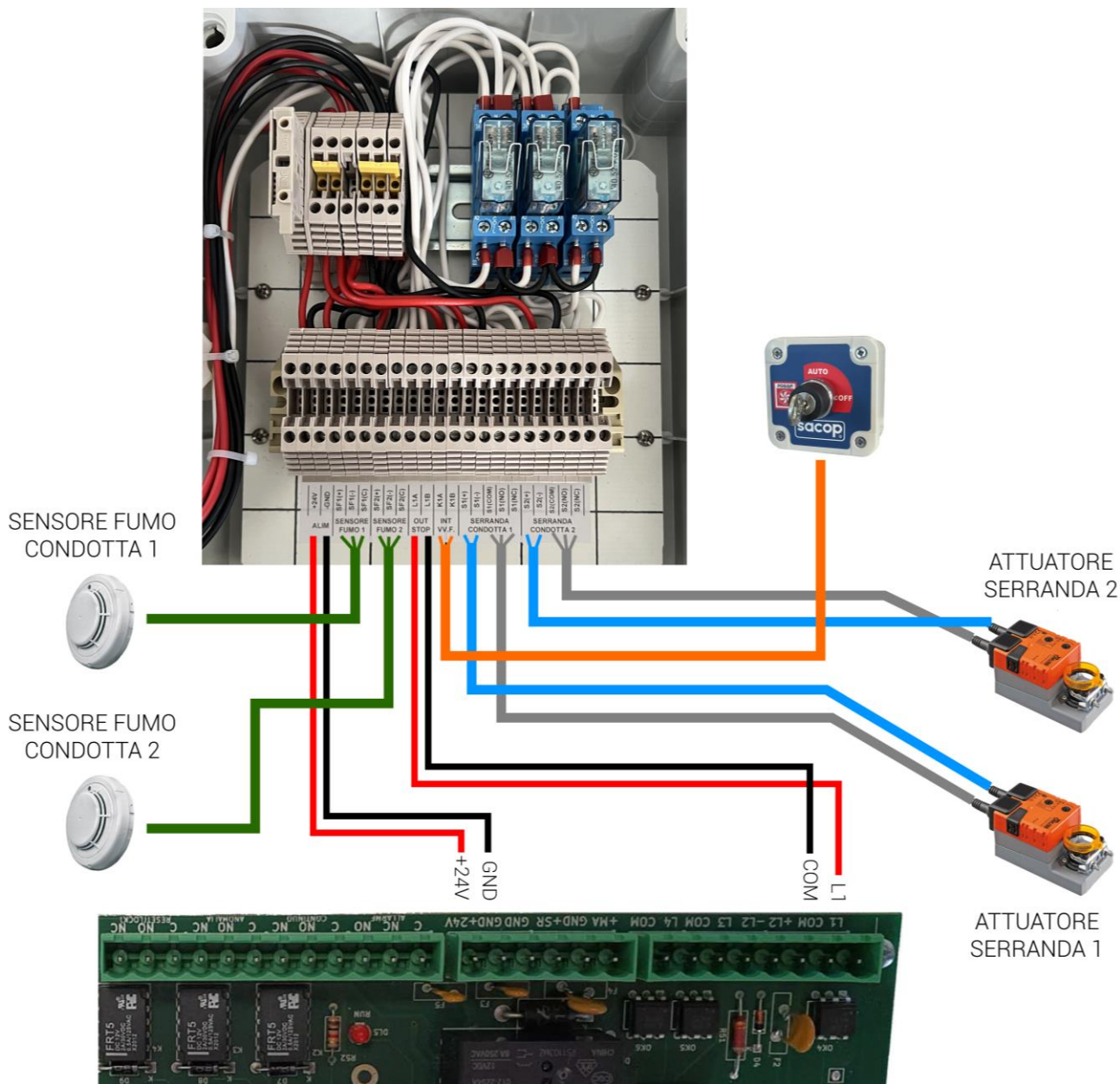
Figura 65 - Schema di collegamento elettrico quadro interfaccia Sacop serrande e pulsante VV.F.
