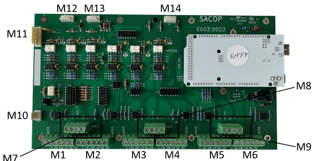
Figura 14 - Morsettiera scheda elettronica Multimaster E003.0022
