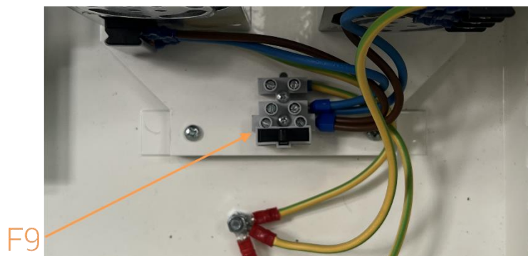
Figura 51 - Fusibile su morsetto di alimentazione unità Multimaster 4
