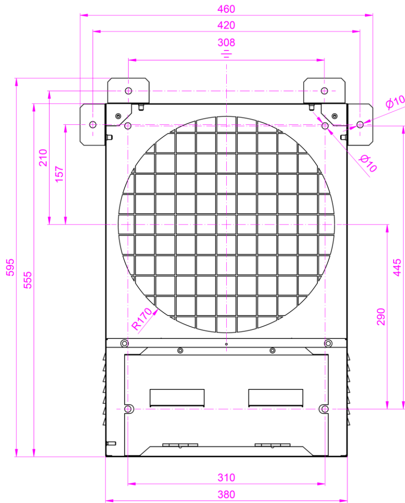
Figura 34 - Quote fori unità Black EVO (valido per tutte le taglie)
