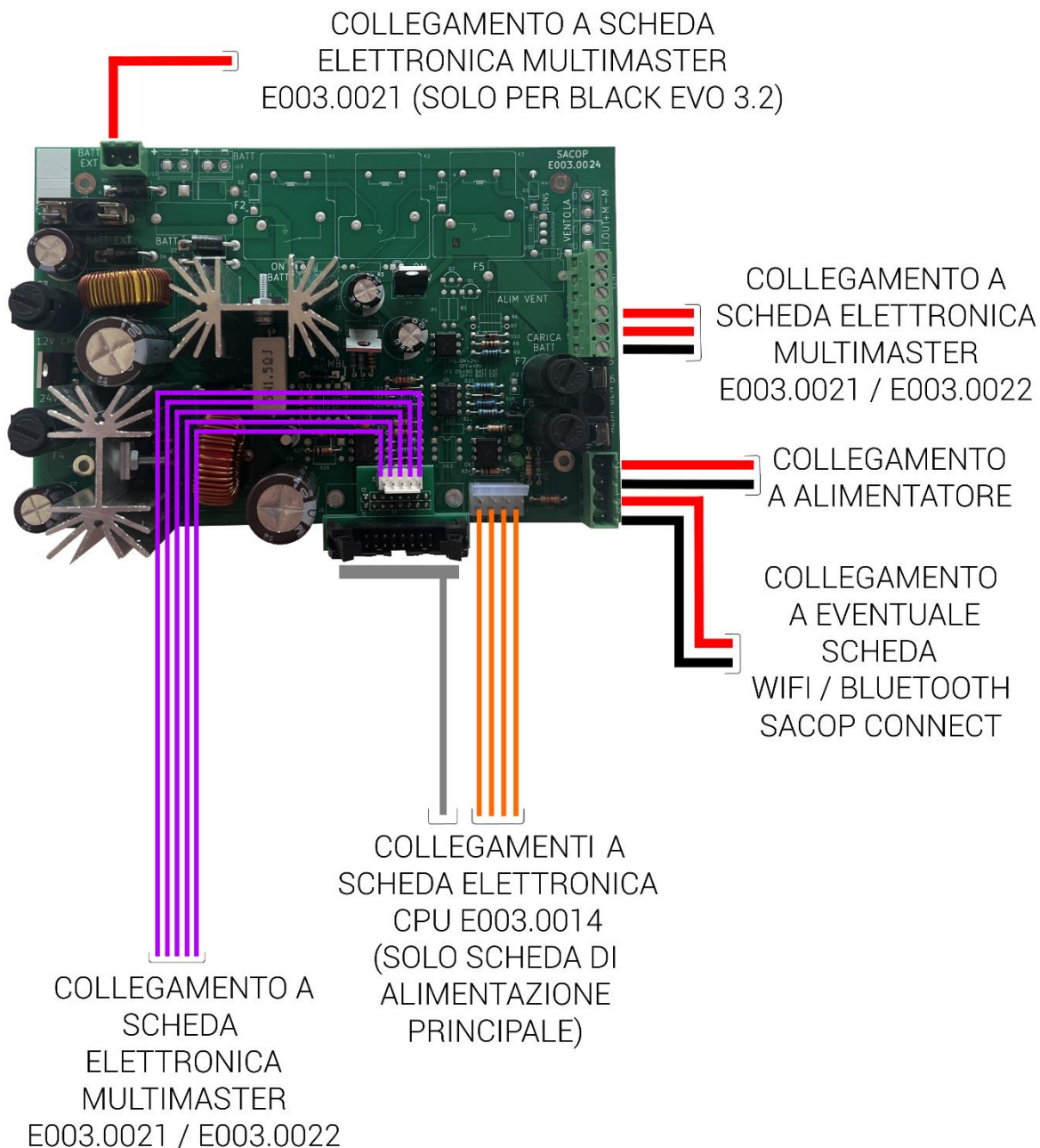
Figura 60 - Schema collegamento elettrico scheda elettronica di alimentazione principale E003.0024 unità Multimaster
