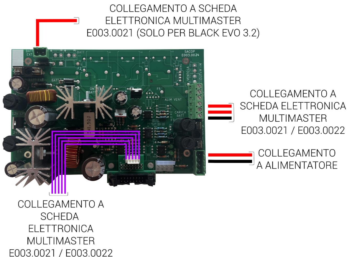
Figura 61 - Schema collegamento elettrico schede elettroniche di alimentazione E003.0024 n.2 e n.3 unità Multimaster
