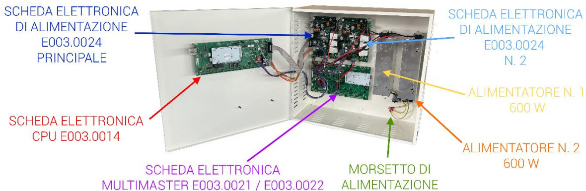
Figura 2 - Componenti principali unità Multimaster 4
