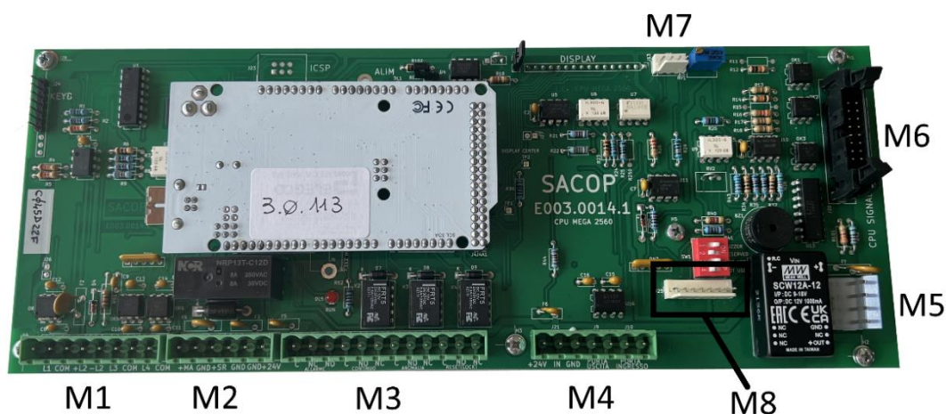
Figura 9 - Morsettiera scheda elettronica CPU E003.0014
