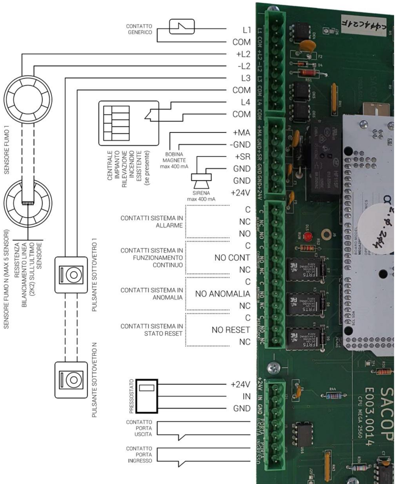
Figura 59 - Schema collegamento elettrico scheda elettronica CPU E003.0014 unità Multimaster - valido per tutti i modelli
