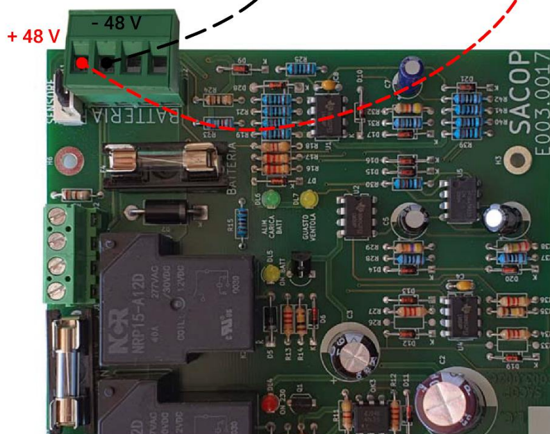
Figura 68 - Schema collegamento batterie unità Black EVO - valido per modello 4.2 (48 V)
