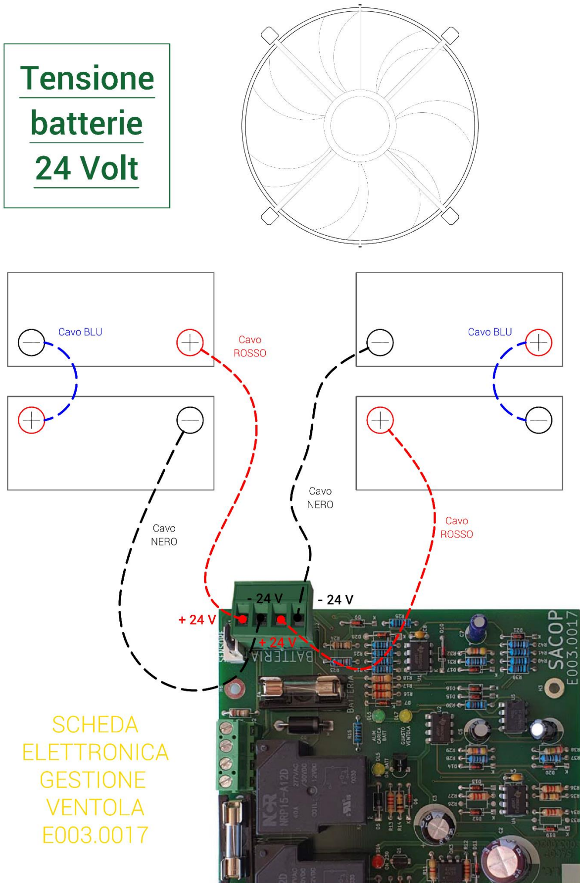
Figura 67 - Schema collegamento batterie unità Black EVO - valido per modello 3.2 (24 V)
