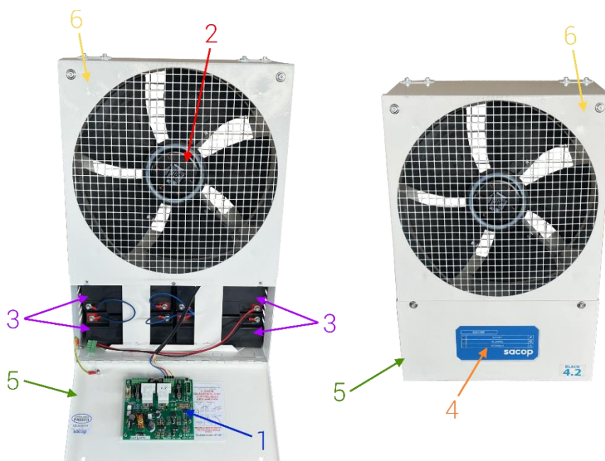
Figura 48 - Indicazione ricambi unità Black EVO 4.2
