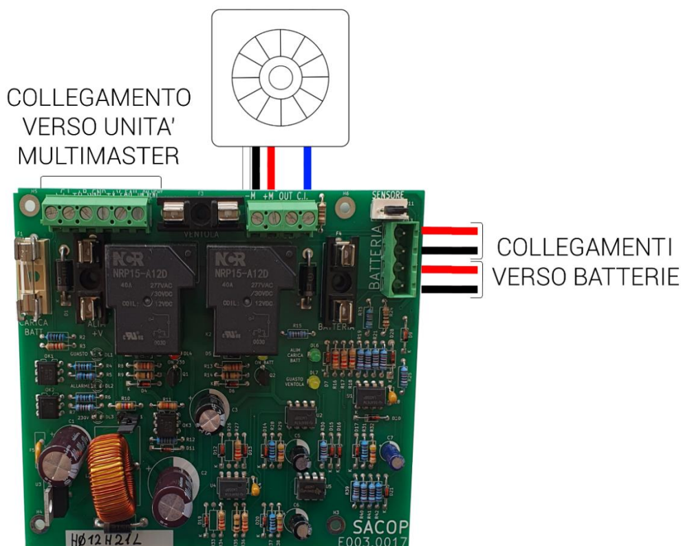
Figura 62 - Schema collegamento elettrico scheda elettronica gestione ventola E003.0017 unità Black EVO 3.2
