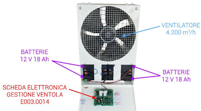
Figura 5 - Componenti principali unità Black EVO 4.2
