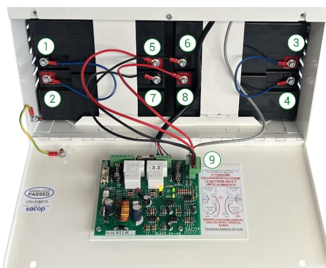
Figura 37 - Foto interna unità Black EVO 3.2 e sequenza operazioni per collegamento cavi batterie
