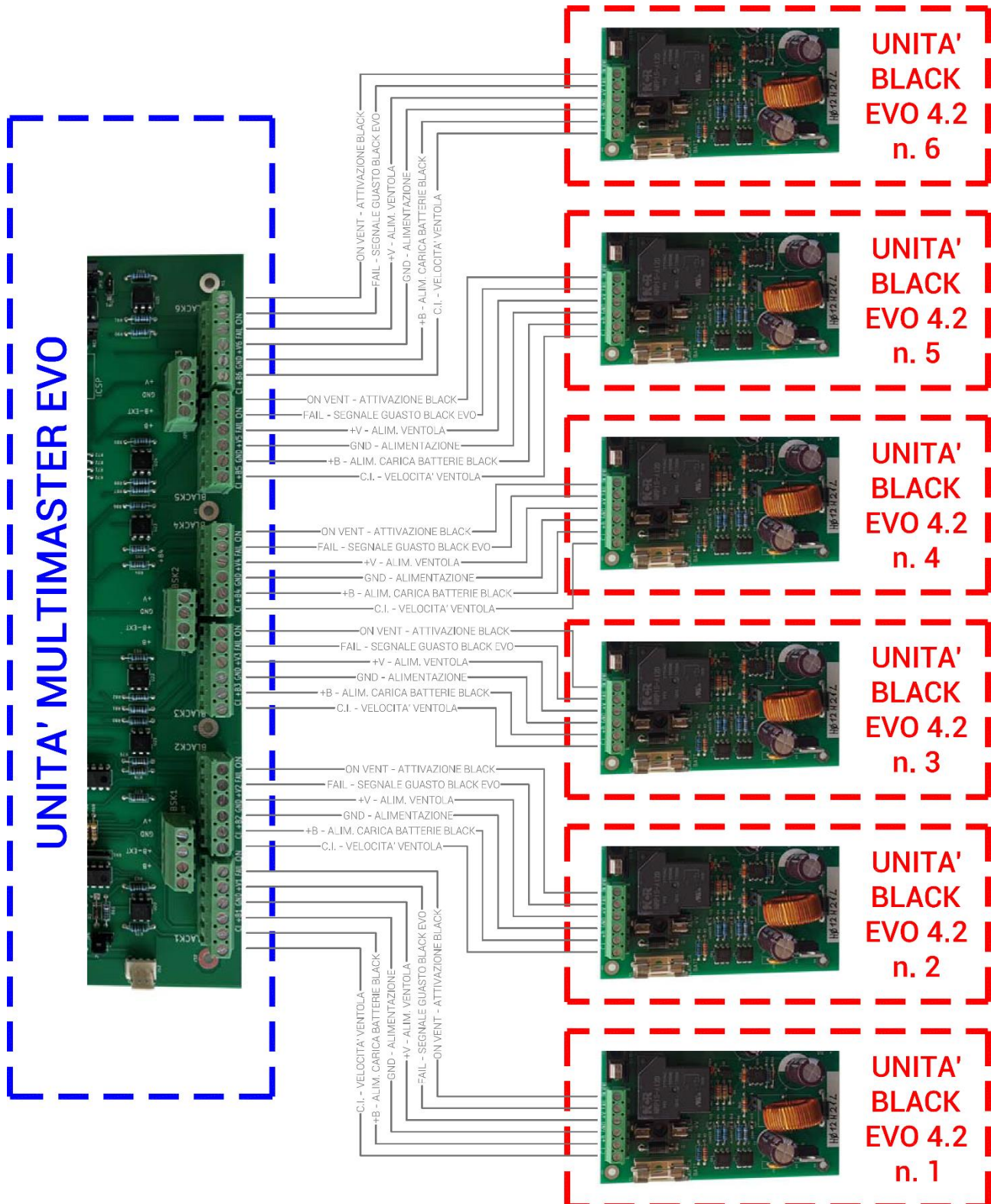
Figura 56 - Schema collegamento elettrico tra scheda elettronica Multimaster E003.0021 / E003.0022 (unità Multimaster) e schede elettroniche gestione ventola E003.0017 (unità Black EVO 4.2)
